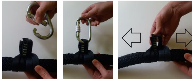
(Prusikknoten)
